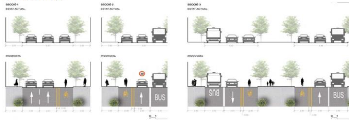
Exemple de proposta tècnica d'ubicacions i amplades de les actuacions tàctiques: Proposta de seccions
